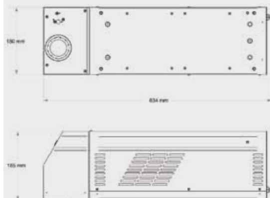
REZONATOR
