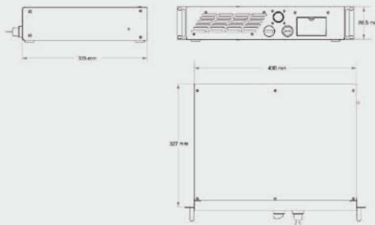
Kontroler
